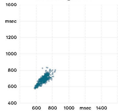
Streudiagramm
