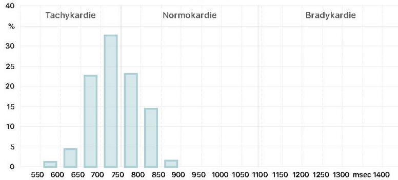
Histogramm
