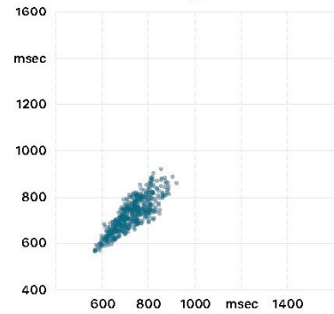
Streudiagramm
