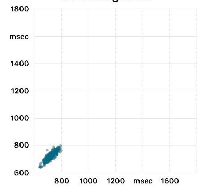
Streudiagramm
