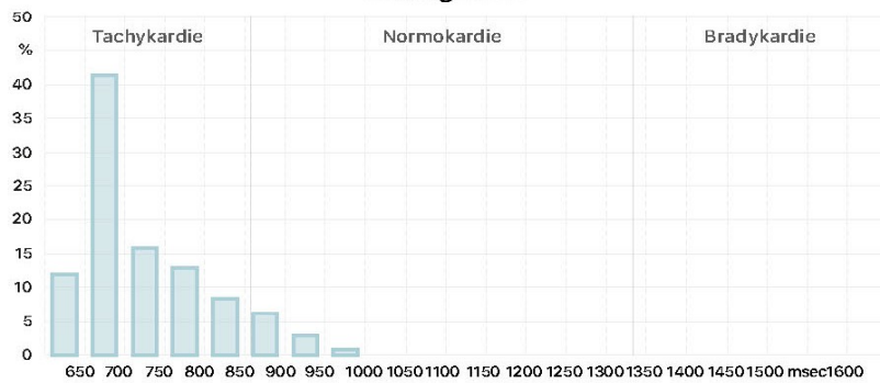
Histogramm
