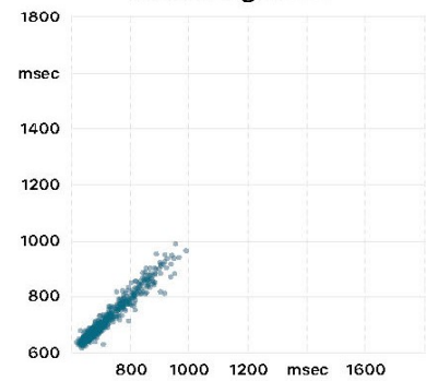
Streudiagramm
