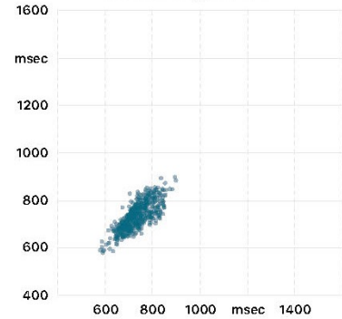
Streudiagramm
