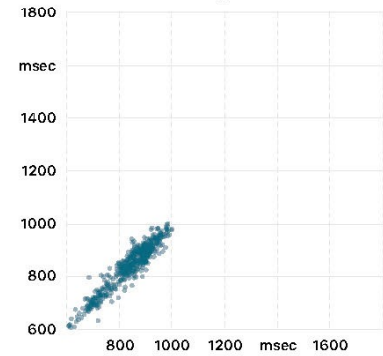
Streudiagramm
