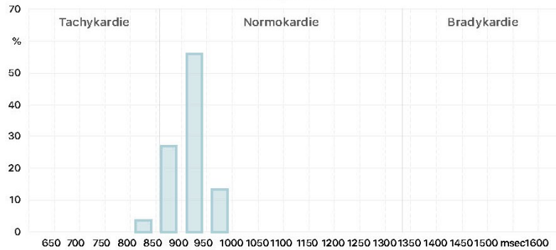
Histogramm
