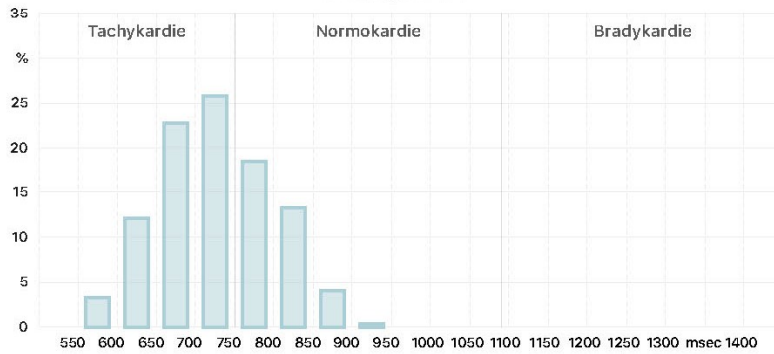
Histogramm
