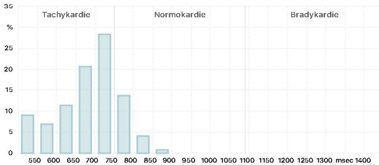
Histogramm
