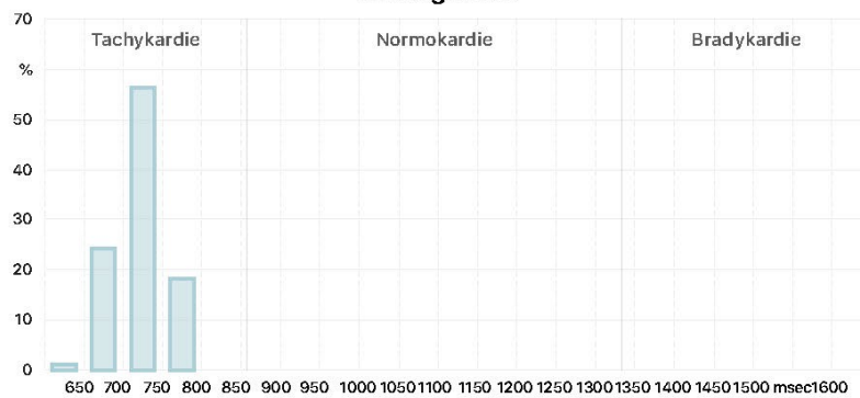
Histogramm
