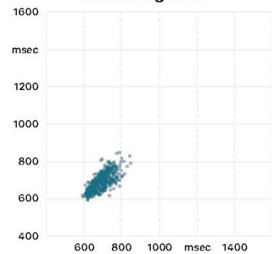
Streudiagramm
