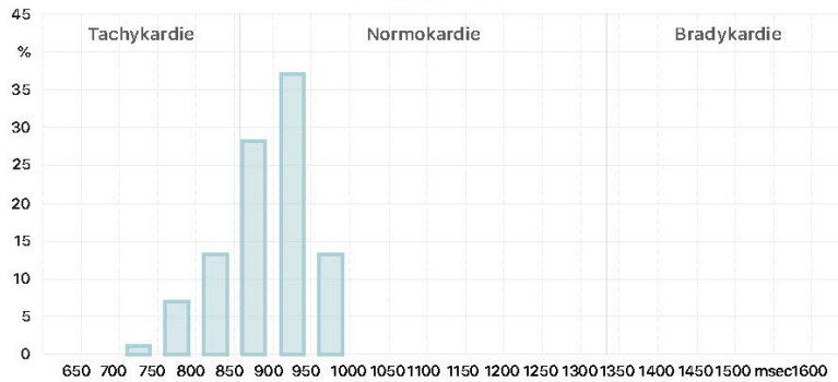
Histogramm
