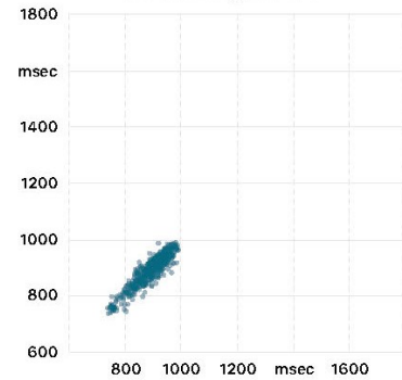
Streudiagramm
