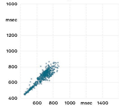
Streudiagramm
