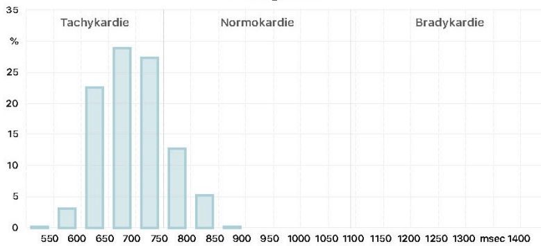
Histogramm
