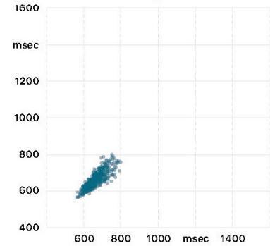
Streudiagramm
