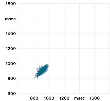
Streudiagramm
