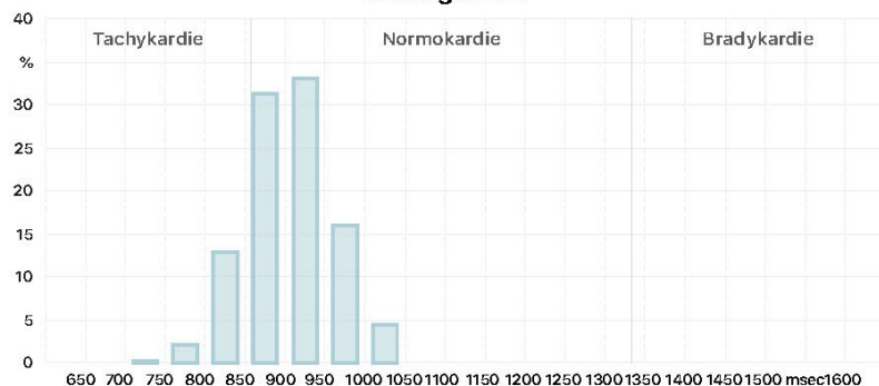
Histogramm
